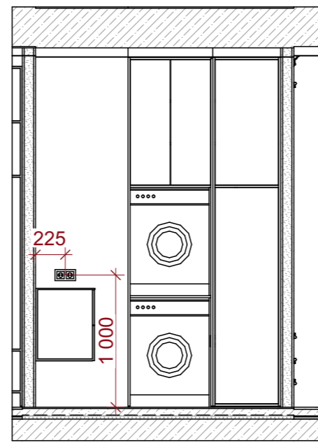
Развертка -П2
