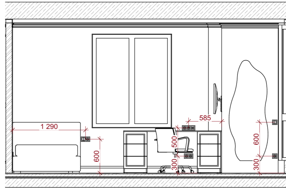
Развертка -СП2
