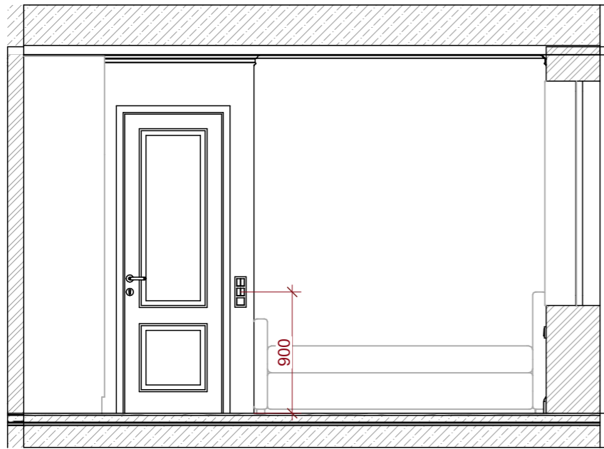
Развертка -СП1
