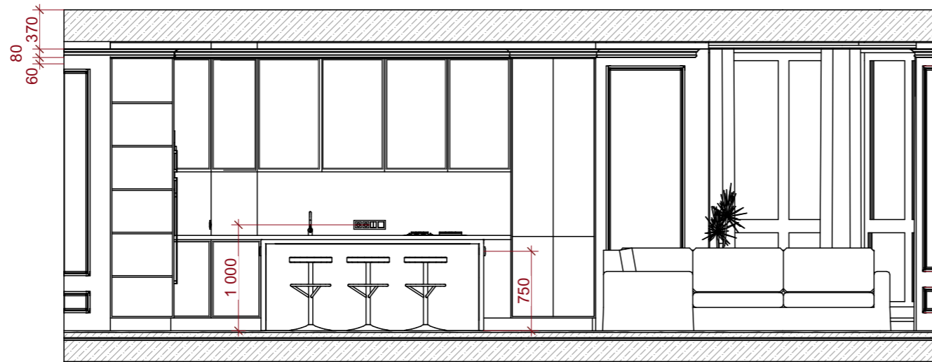
Развертка -К3
