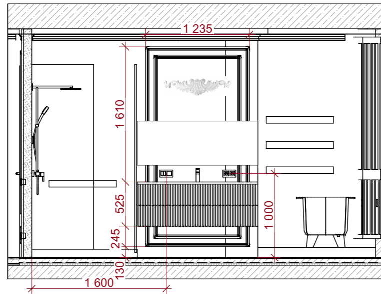
Развертка -В2
