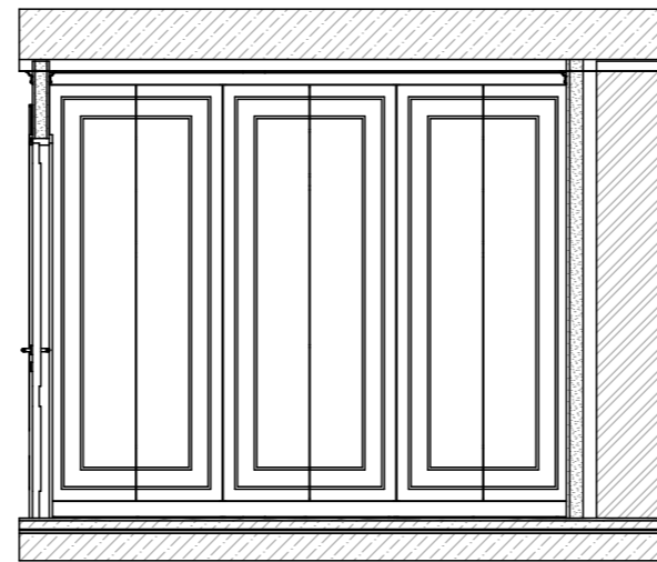
Развертка -С2
