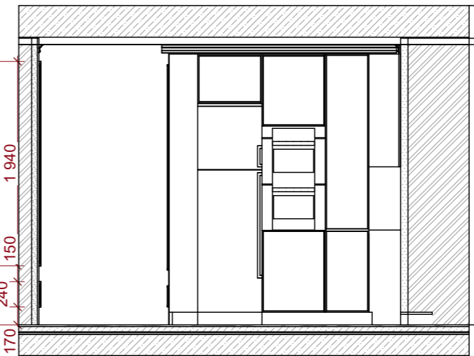
Развертка -К4
