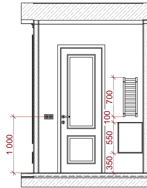
Развертка -П4
