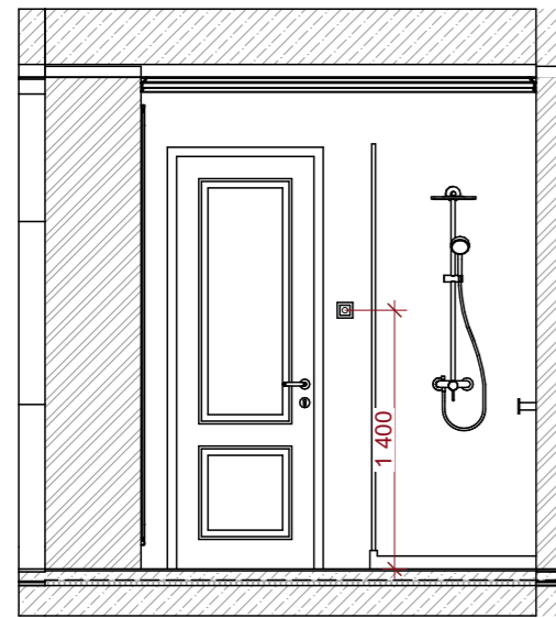
Развертка -В1
