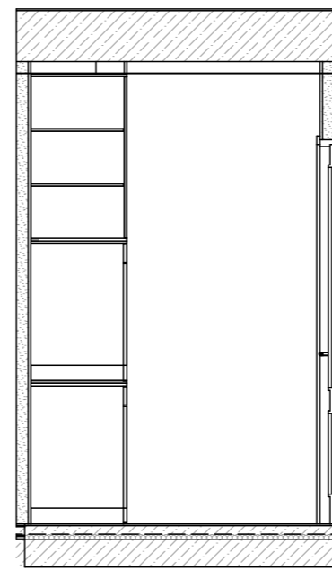
Развертка -П3
