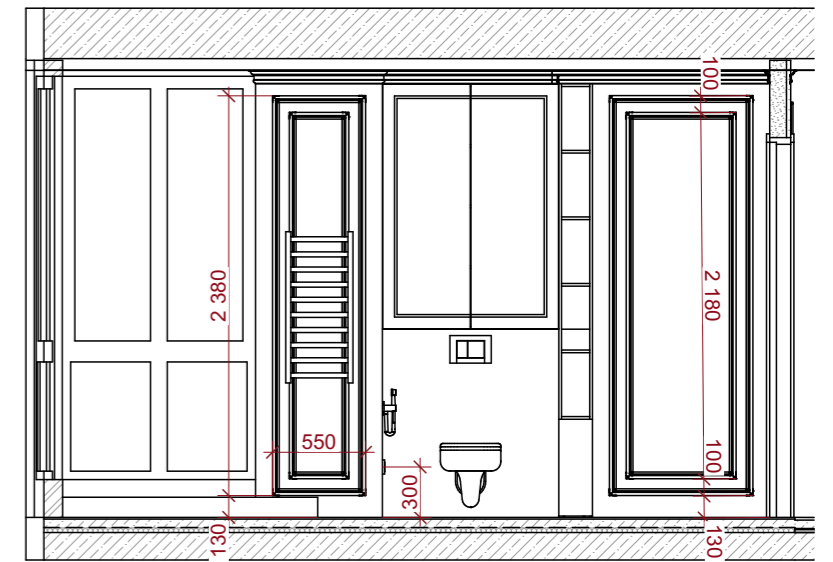
Развертка -В4
