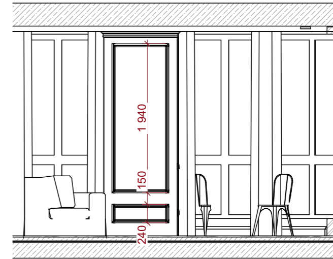
Развертка -К2
