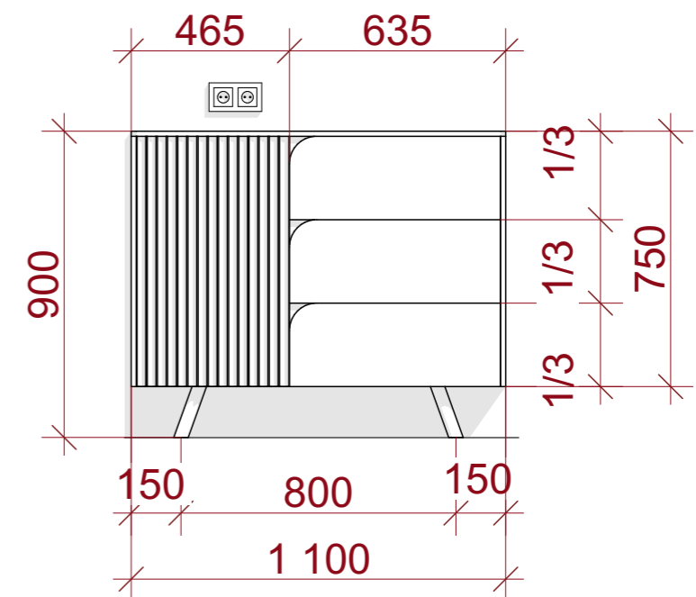
Вид спереди
